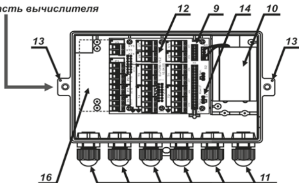
Электронный модуль вычислителя
